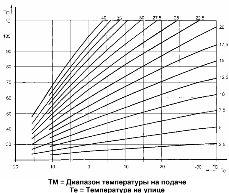
Рис. 11: Выбор рабочей кривой датчика уличной температуры при наличии климатического регулятора QAA 73
